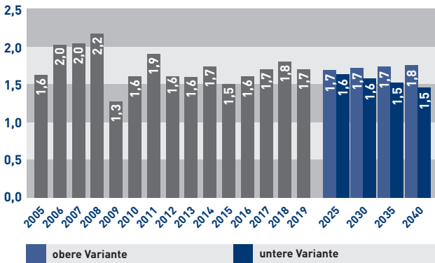
Abb. 45: Produktionsmenge von Gießereialsanden (in Mio. t)
