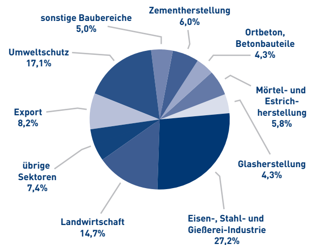
Abb. 19: Verwendung von Kalk- und Dolomitstein für ungebrannte Produkte, Steine/Steinmehl* 2019
